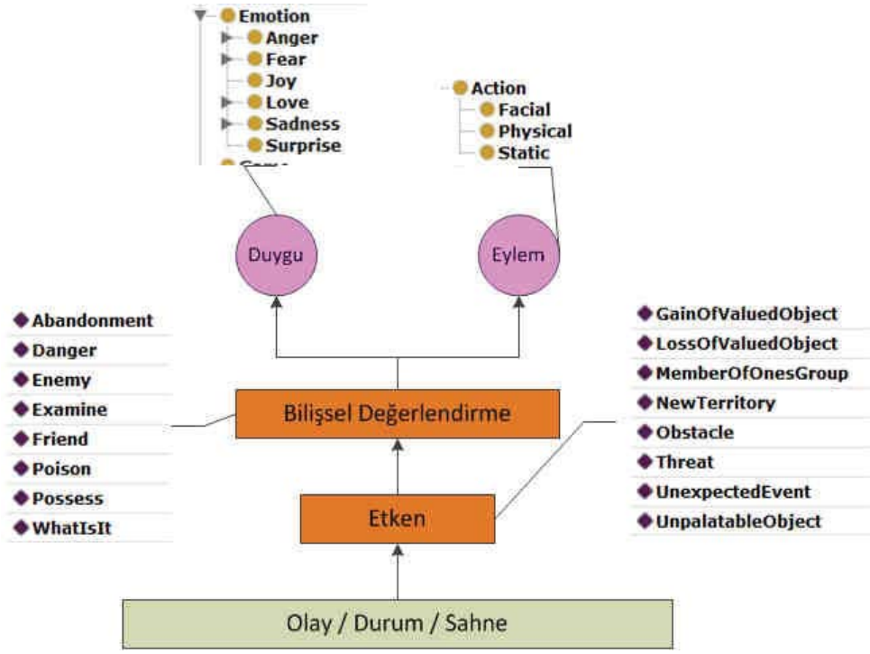
Şekil 4. Sistemin Dört Temel Bileşeni
