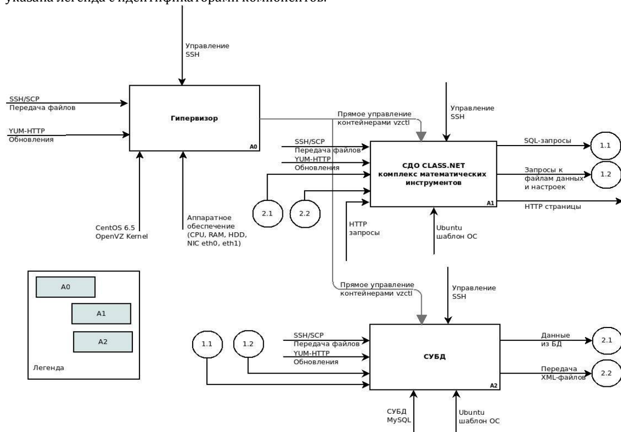
Рис.2. Модель связей СДО CLASS.NET
