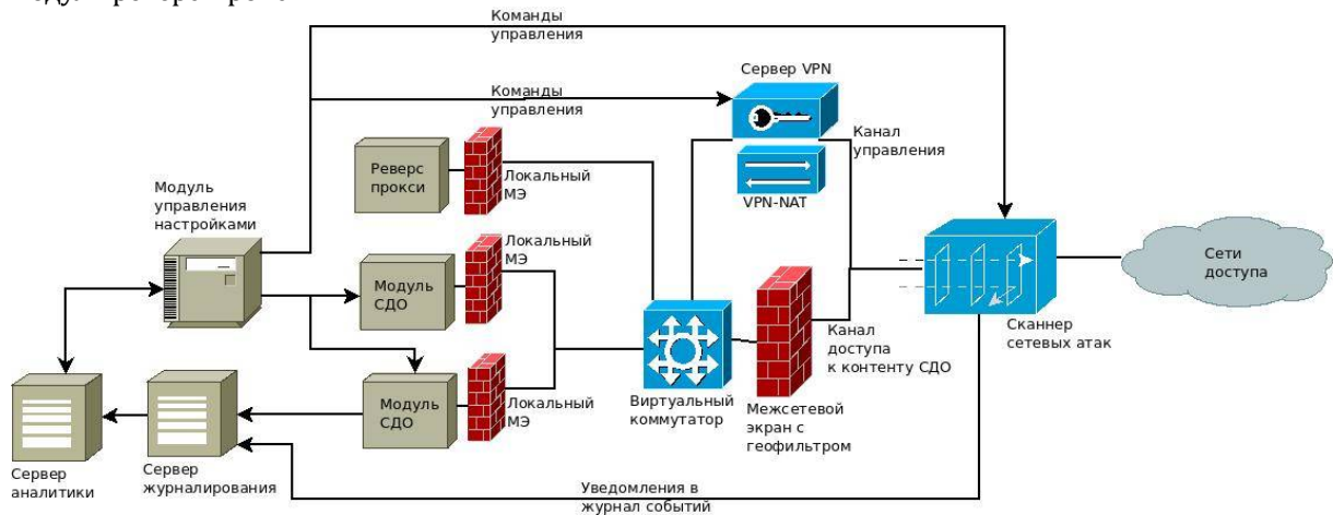
Рис.3. Схема сети СДО CLASS.NET и каналов передачи служебных сигналов
