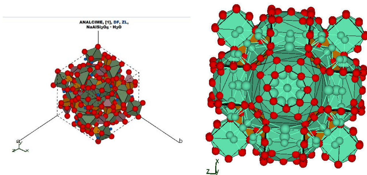
Рис. 1. Примеры интерактивных моделей кристаллической структуры (смешанное представление в шарах и полиэдрах)
