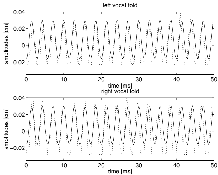
Abb. 1. Ergebnis der Approximation (durchgezogene Linien) an gesunde Stimmlippenbewegung (gestrichelt) in einem Zeitfenster von 50 \text{ ms} . Das obere Bild entspricht der linken und das untere der rechten Seite der Stimmlippen.
