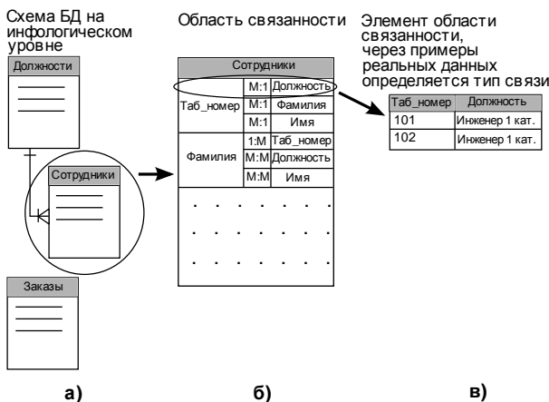
Рис. 2. Определение связи между атрибутами Tab_Номер и Должность через использование двухстрочного отношения: а) схема БД на инфологическом уровне; б) детализирована область связанности Сотрудники ; в) детализирован элемент связанности Tab_Номер – Должность области связанности Сотрудники , связь между атрибутами которого определяется через использование двухстрочного отношения, заполненного реальными данными
