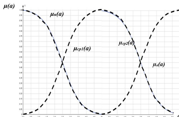
Рис. 4. Функции принадлежности \mu(a) экспертных оценок метапредметных образовательных результатов для низкого, среднего и высокого уровня развития компетенций
