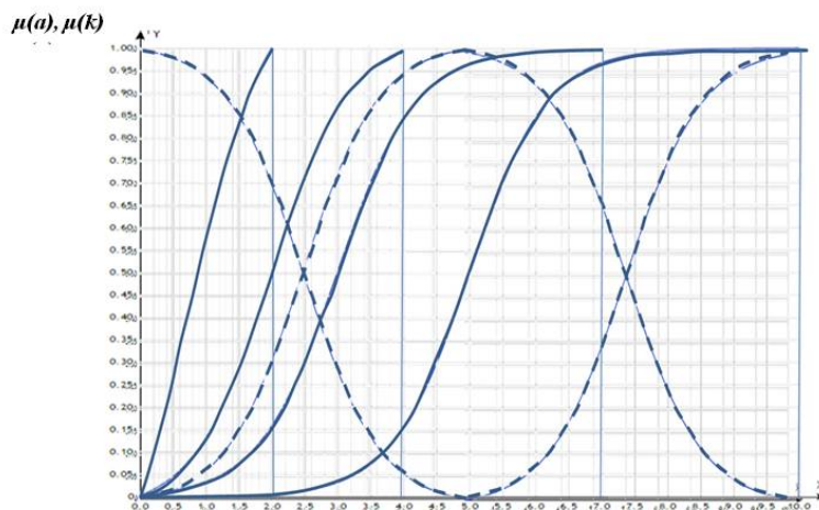
Рис. 5. Наложение функций принадлежности \mu(k) (сплошные линии) и \mu(a) (пунктир) в интервале единой шкалы оценок 0-10 для определения результирующей оценки, учитывающей степень достоверности соответствия наборов УУД заданиям \mu(k) и степень достоверности оценки эксперта \mu(a)
