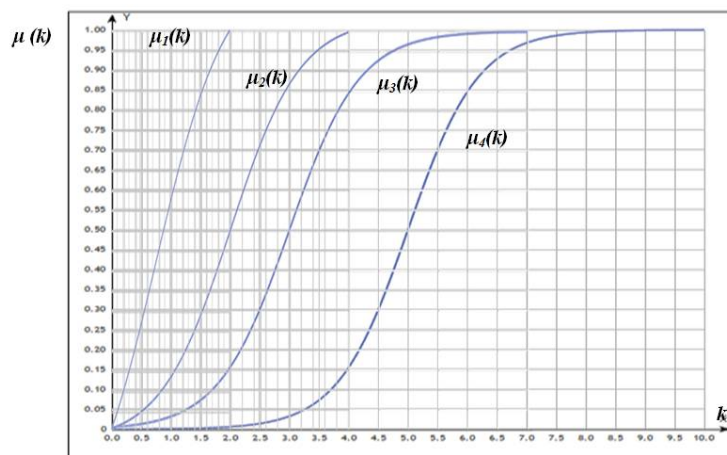
Рис. 3. Зависимость функции принадлежности \mu(k) , определяющей степень соответствия наборов УУД заданиям четырёх интервалов сложности от потенциальных оценок в интервале от 0 до 10
