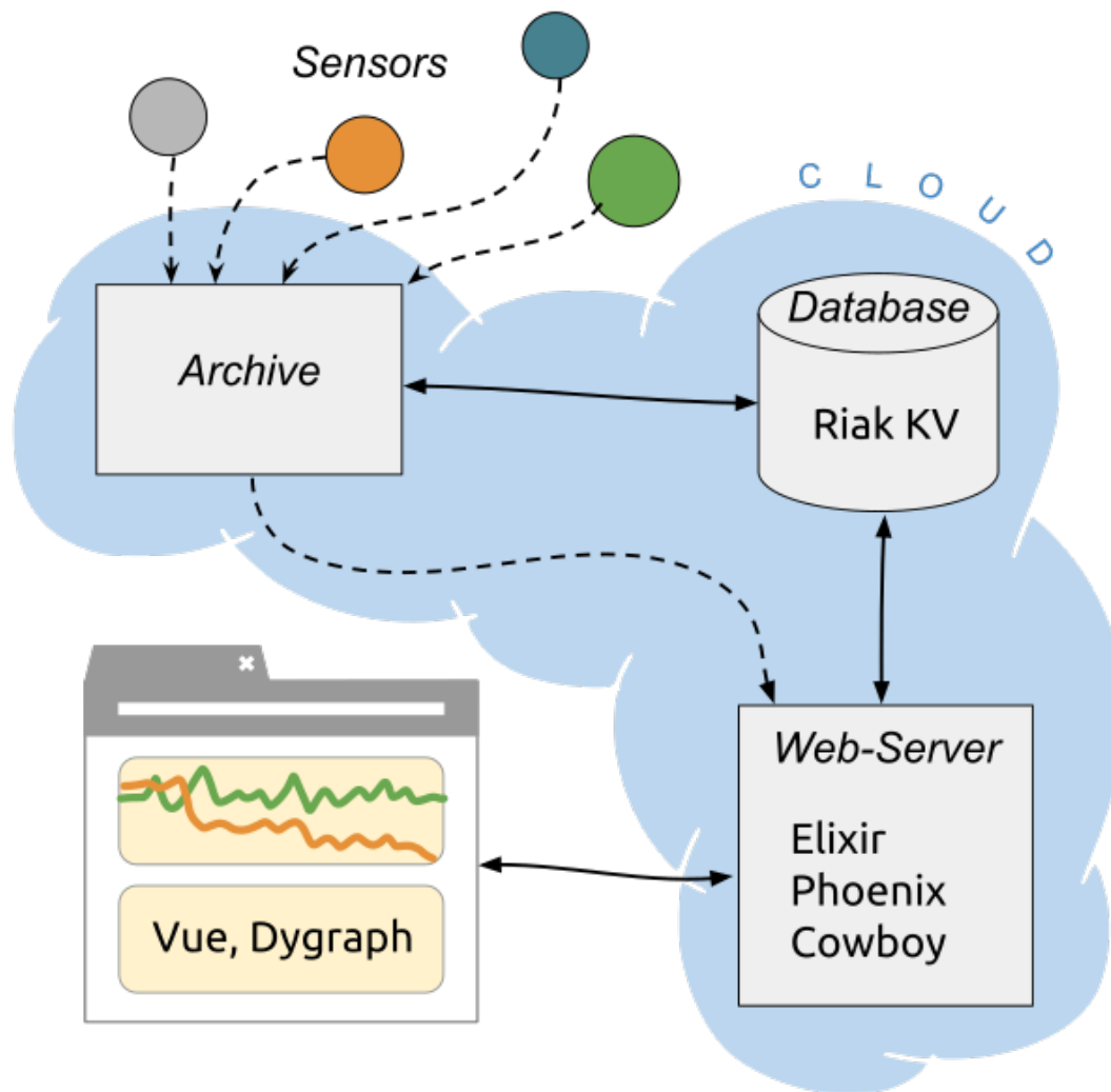
Рис. 1. Обзор архитектуры системы мониторинга
