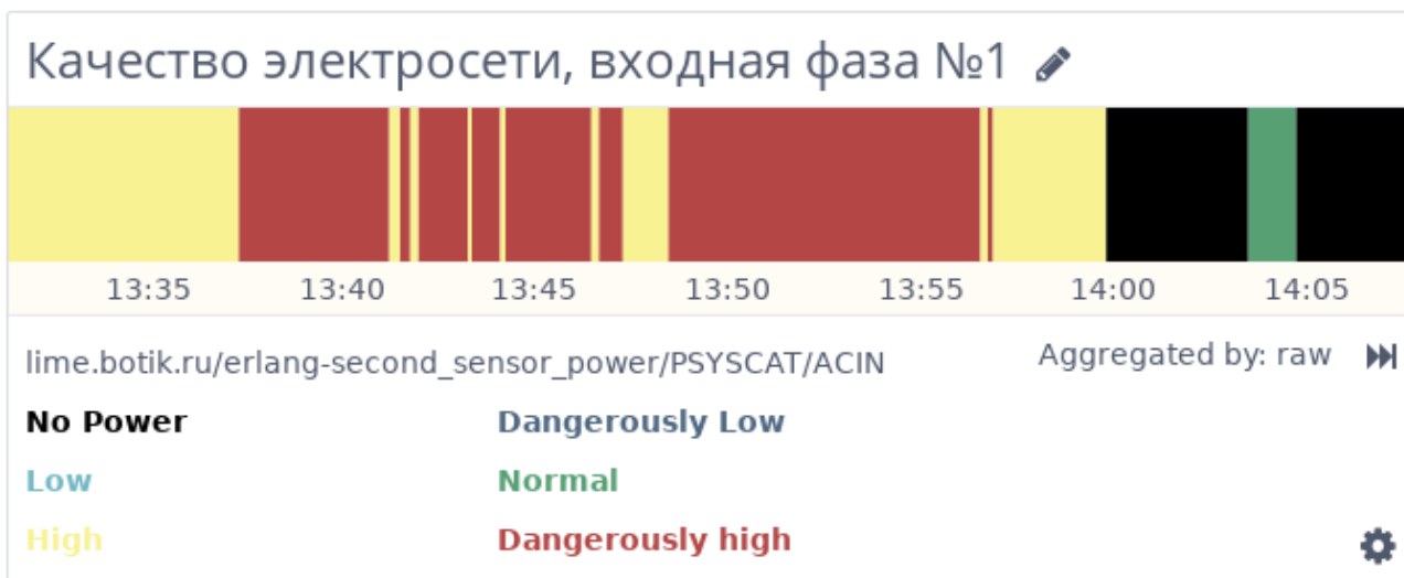
Рис. 4. Пример отображения неагрегированных данных категорий состояния
