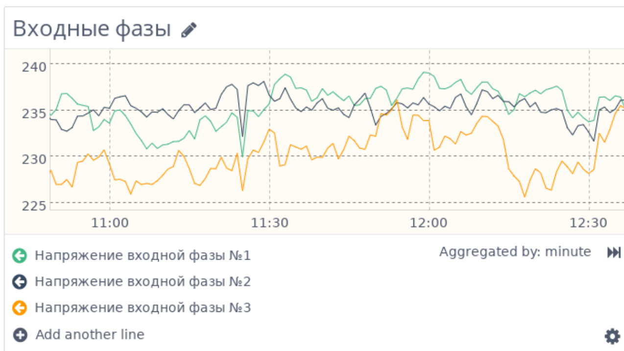
Рис. 2. Пример отображения сенсорных данных графиком
