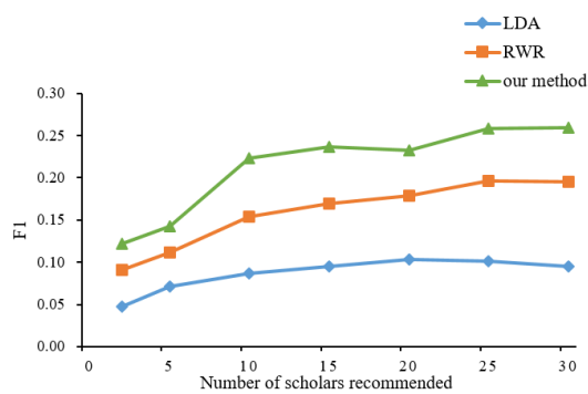
Fig. 6. F1 Score
